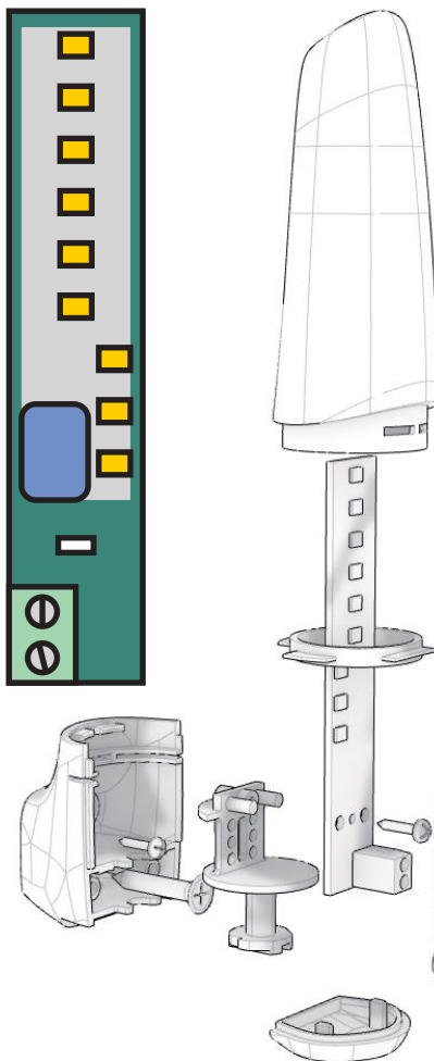
7. UTILIZZANDO UNA MONETA O UN CACCIAVITE ORIENTARE LO STAMPATO. +180° / - 180° di rotazione. Use a coin or a screwdriver to rotate the PCB and adjust the alignment between TX and RX. +180° / - 180° rotation.
